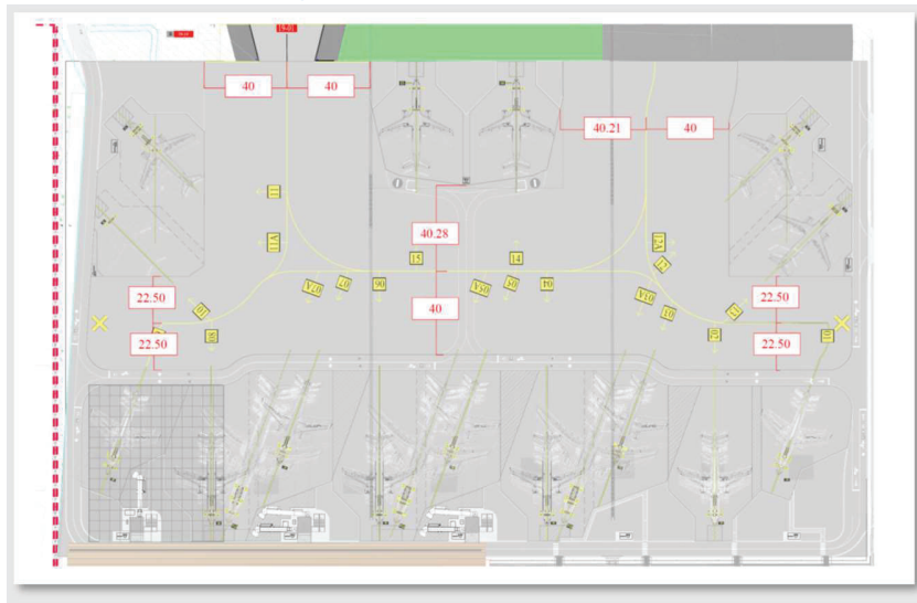
Ilustración 55: Configuración de la ampliación de la Plataforma Principal
