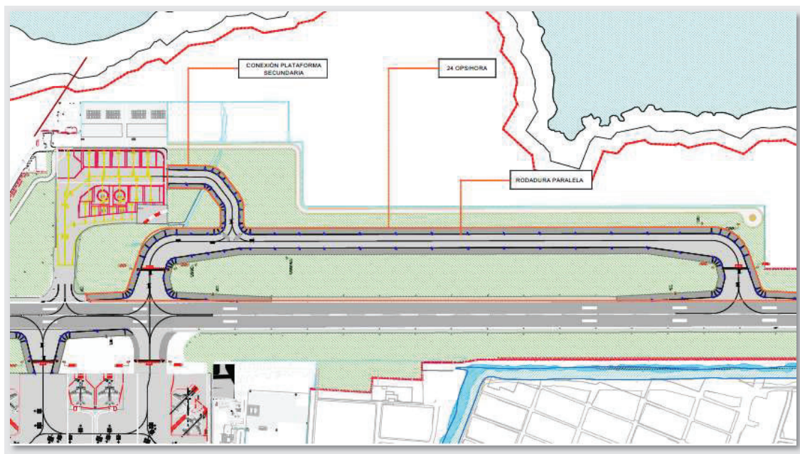
Ilustración 87 Rodadura paralela
