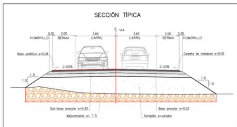
(d) Sección típica de la UF7
