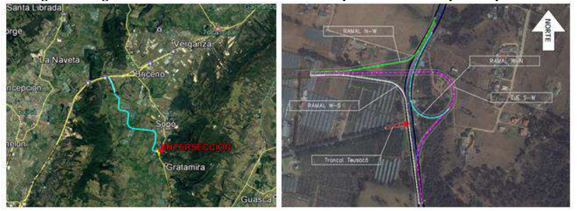
Figura 5 - Figura ilustrativa de la intersección tres esquinas a desnivel tipo trompeta
