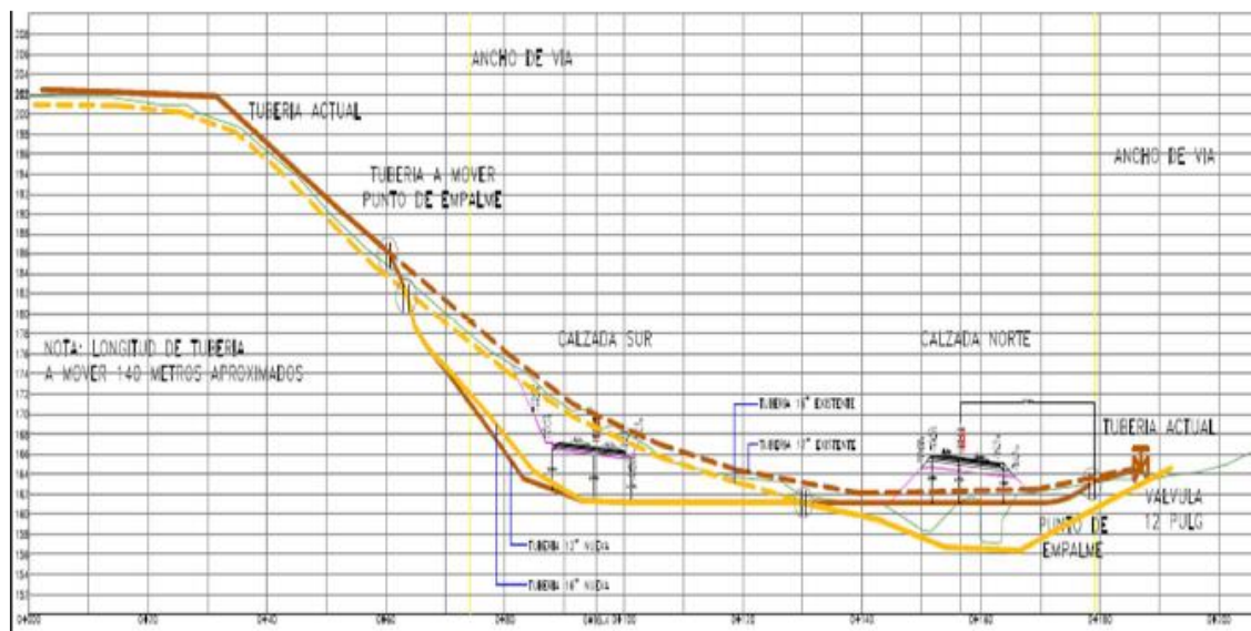
Ilustración 7 Variantes verticales
