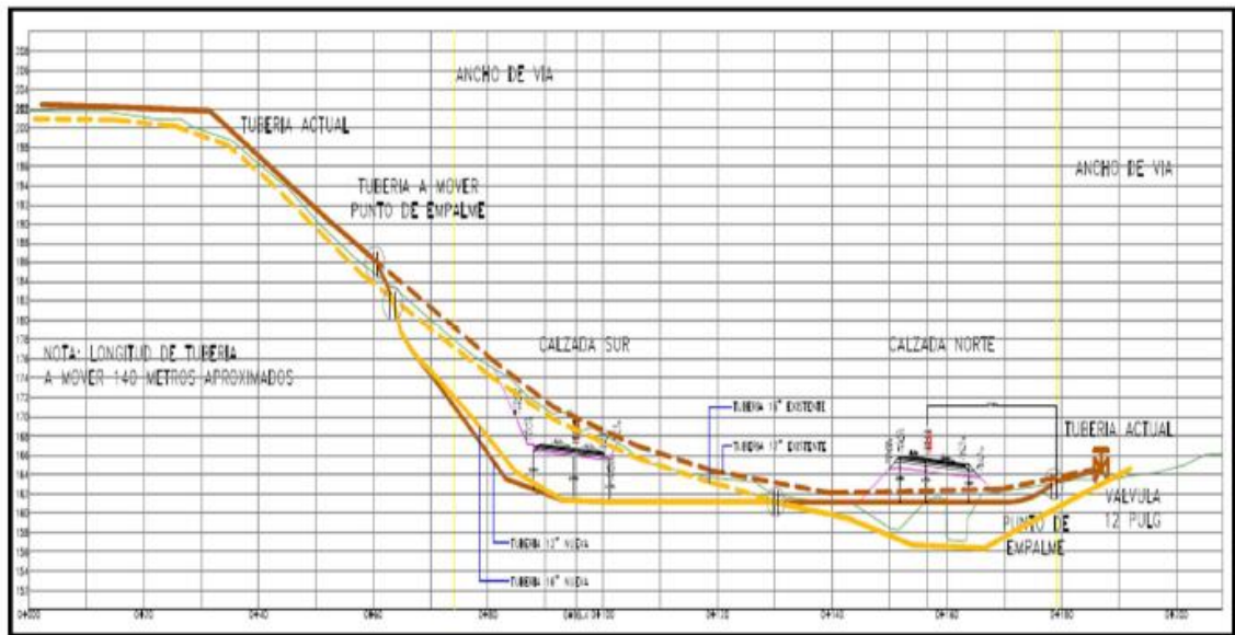
Ilustración 7 Variantes verticales
