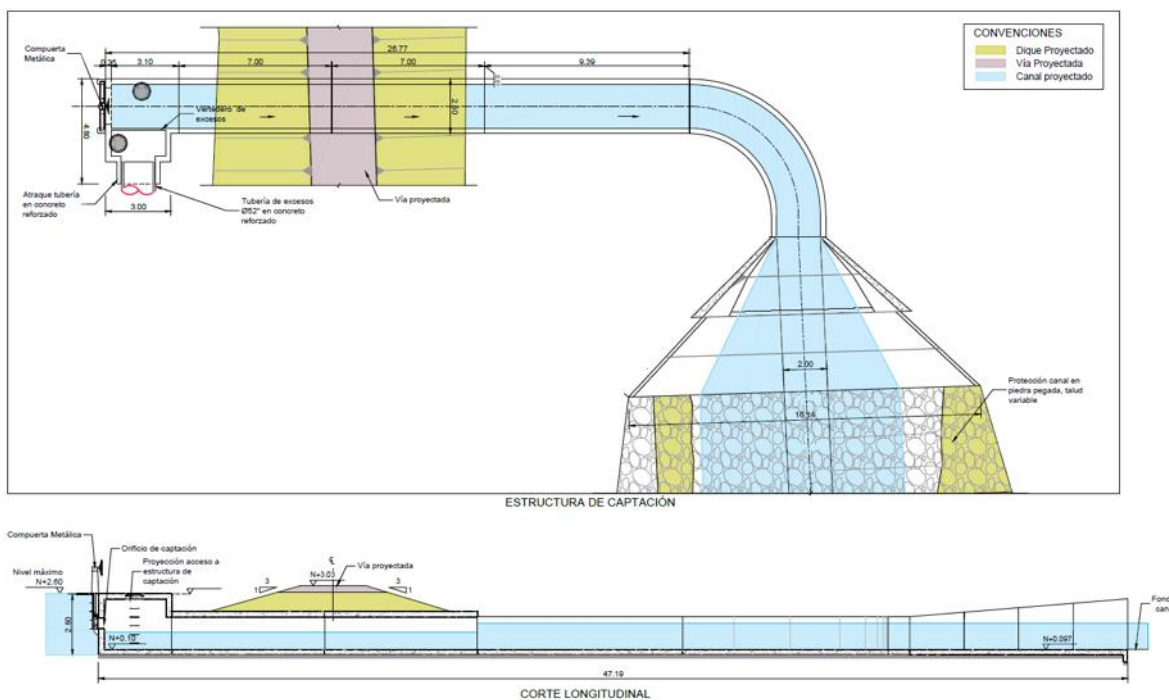
Figura 2-31 Esquemmatización captación de la obra G3 K0+000
