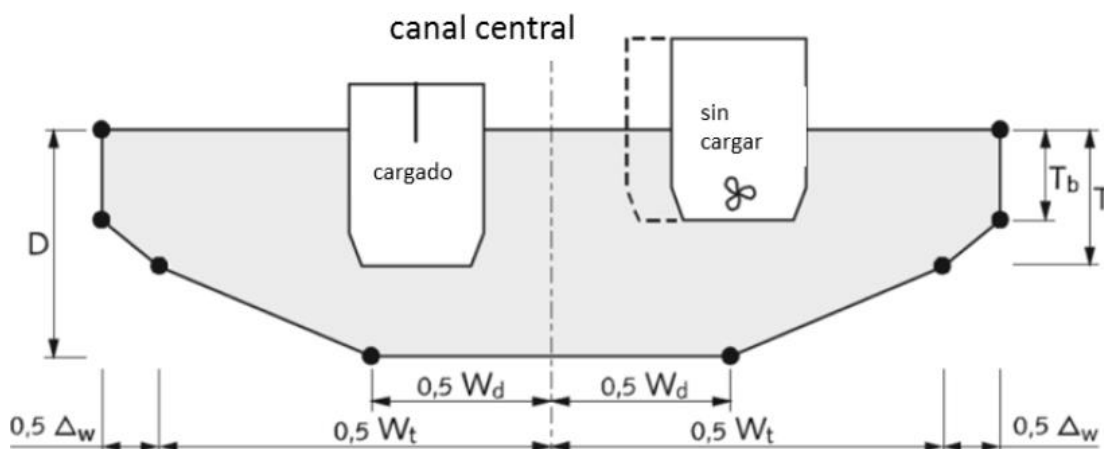
Figura 2-63 Perfil de Canal mínimo para tramos rectos
