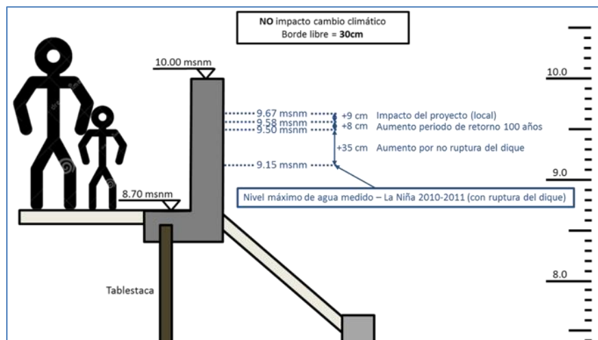
Figura 2-62 Esquematzación del nuevo muro de Calamar (cerca la entrada del Canal del Dique). Segunda etapa.
