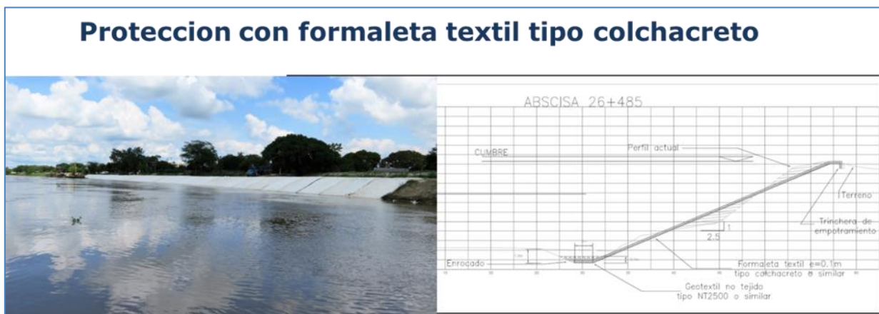
Figura 2-65 Protección de orillas con formaleta textil rellena de concreto y trinchera de empotramiento
