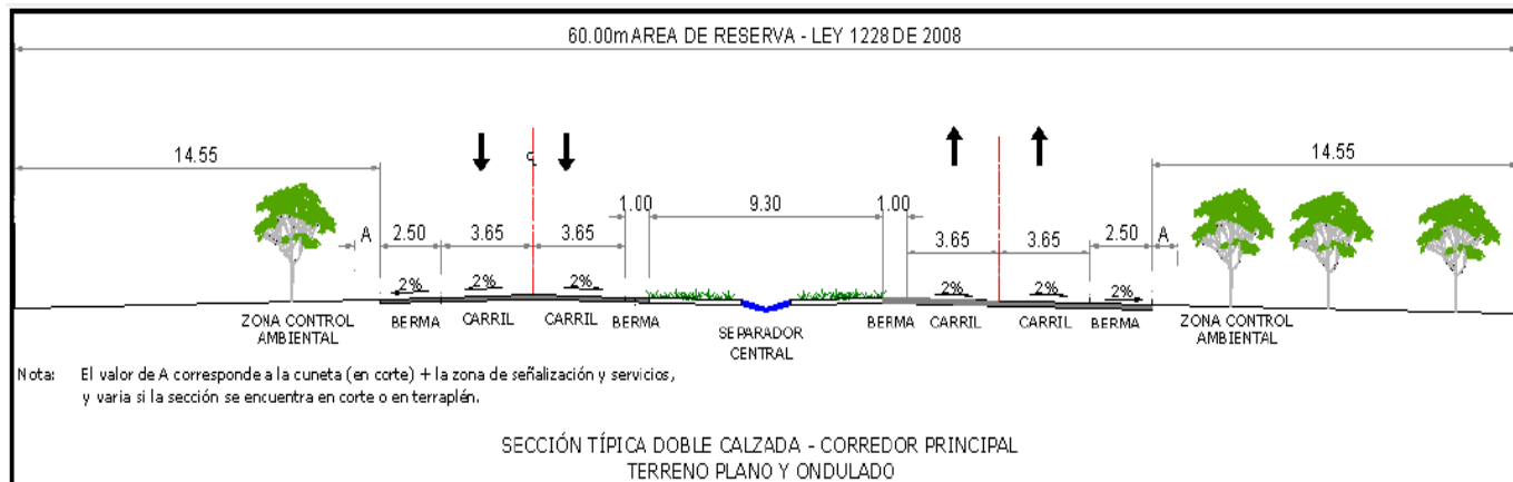
Figura 3 - Sección de la Vía Típica
