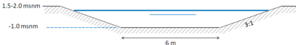
Figura 2-24 Sección transversal de Caño Rico cerca a la entrada
