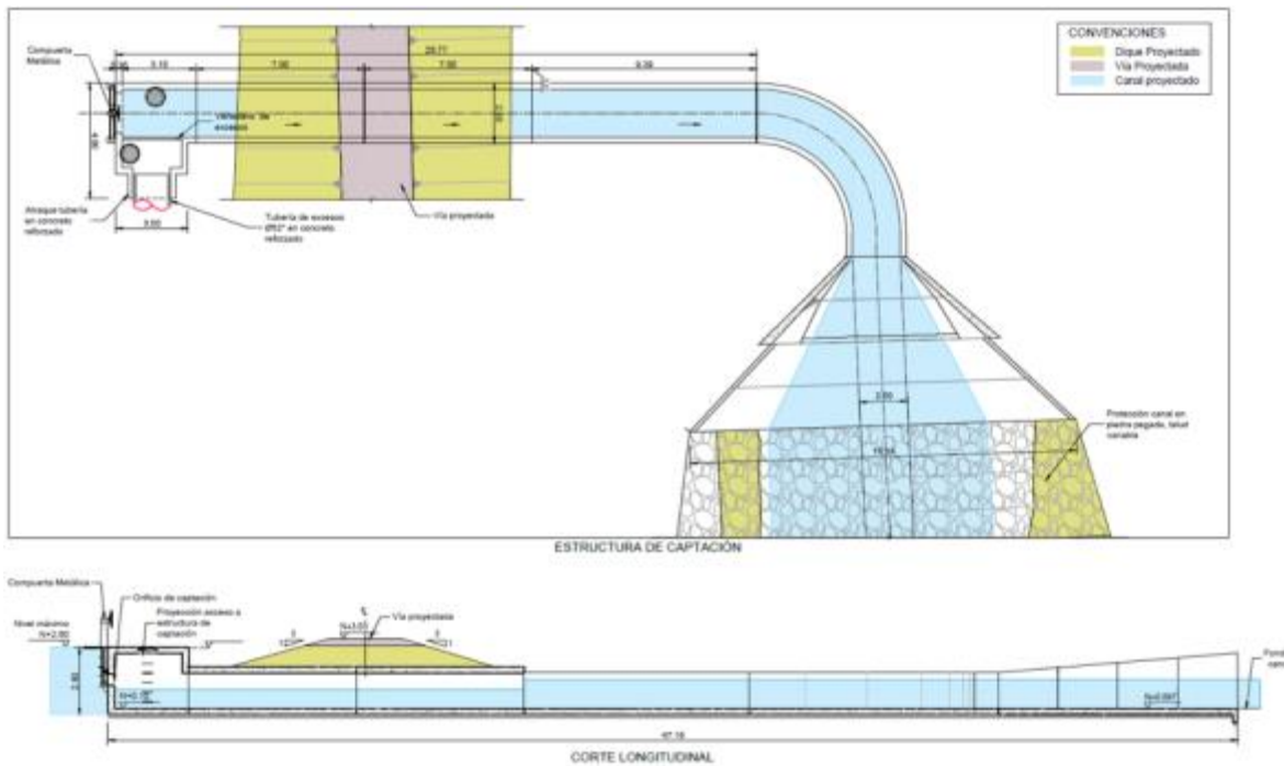
Figura 2-34 Esquemmatización capitación de la obra G3 K0+000
