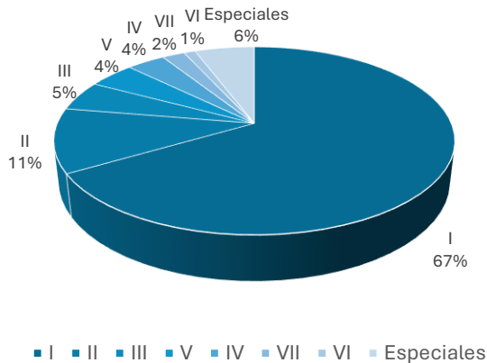
Gráfico 7. Porcentajes de participación del tráfico total por categorías vehiculares en diciembre de 2025 pr
