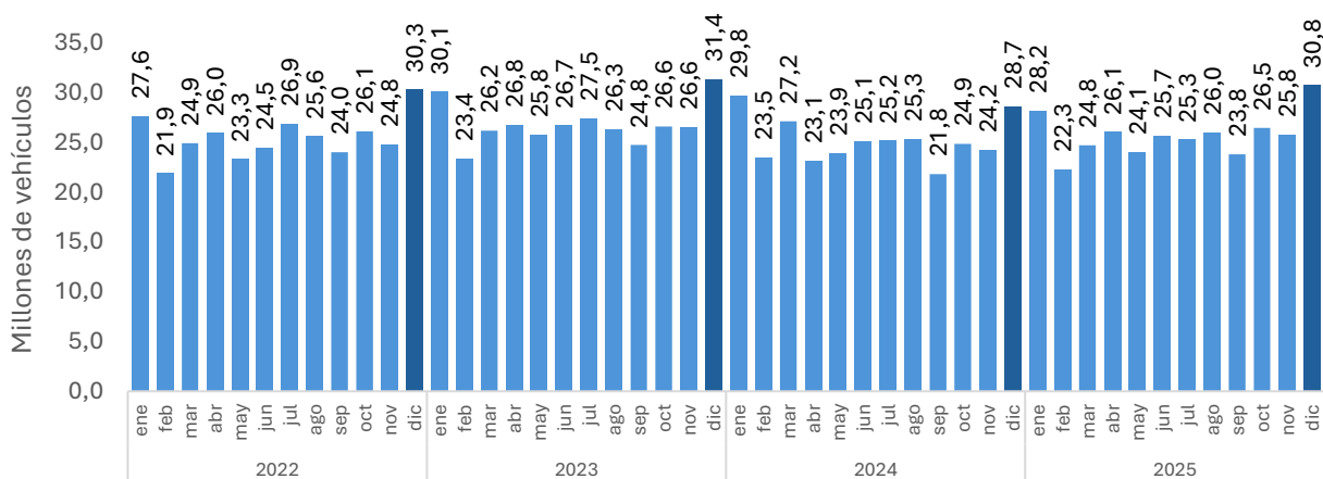
Gráfico 1. Tráfico total mensual - Base de datos acopiada final. Enero 2022 – diciembre de 2025 pr
