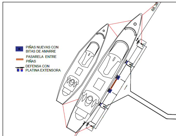
Figura No.4 Atraque simultáneo de 2 motonaves
