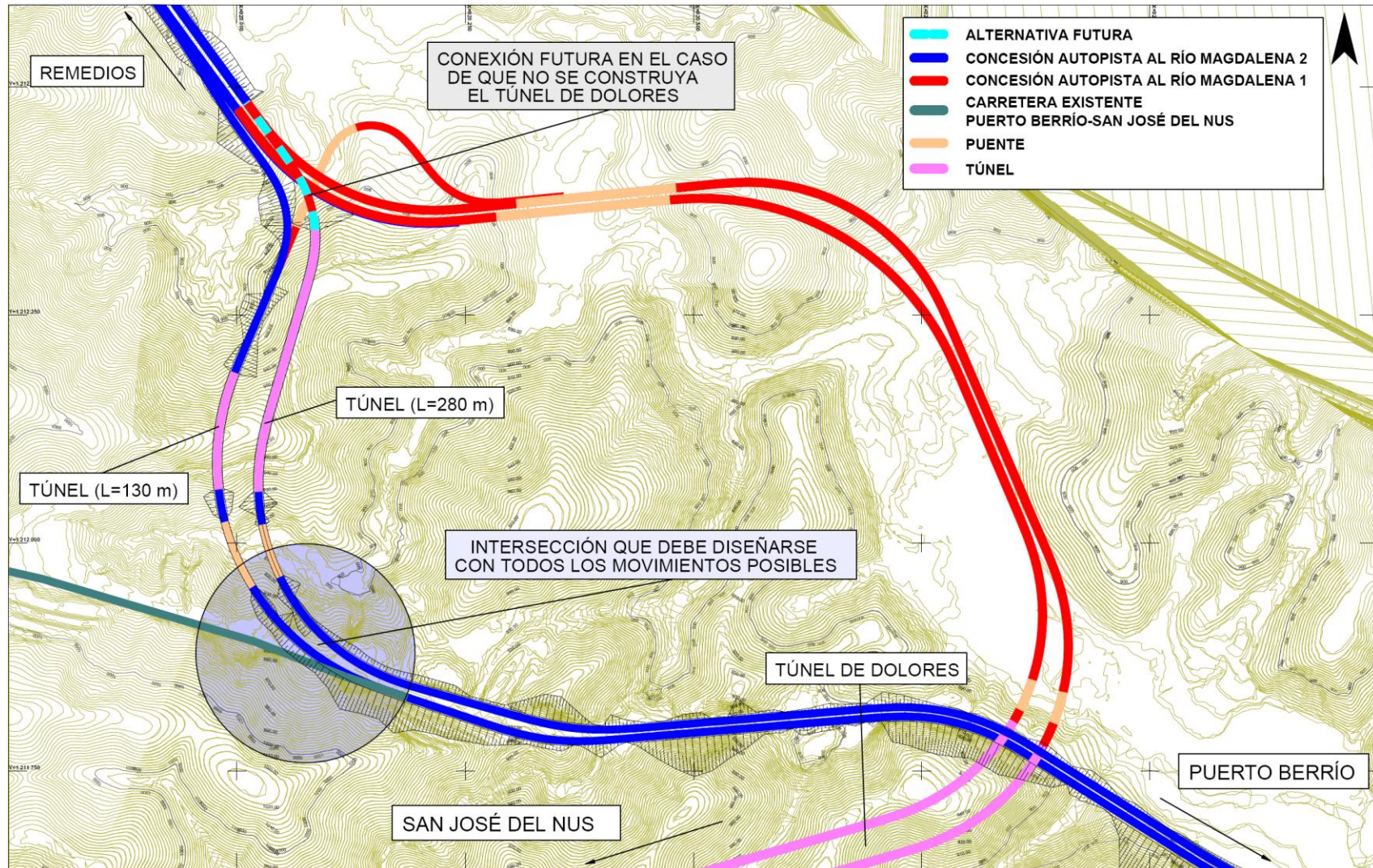
Figura 2 – Esquema de empalmes Alto de Dolores
