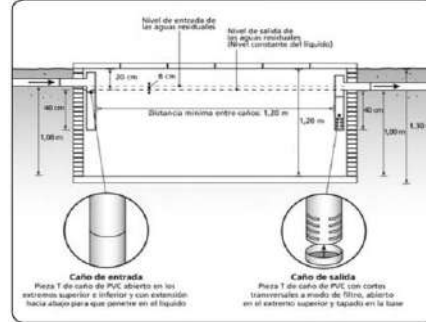
FIGURA 10 - LA CAMARA SÉPTICA - Medidas
