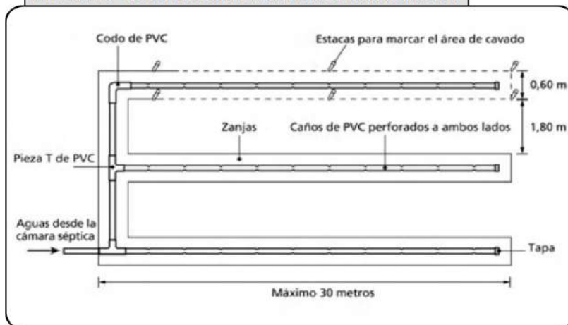
FIGURA 13 - CONSTRUCCIÓN DEL TERRENO DE INFILTRACIÓN
