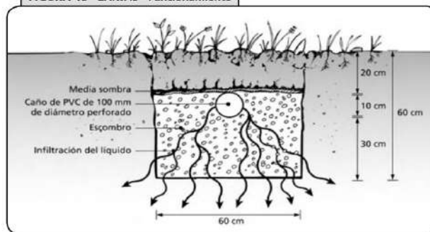
FIGURA 15 - ZANJAS - Funcionamiento
