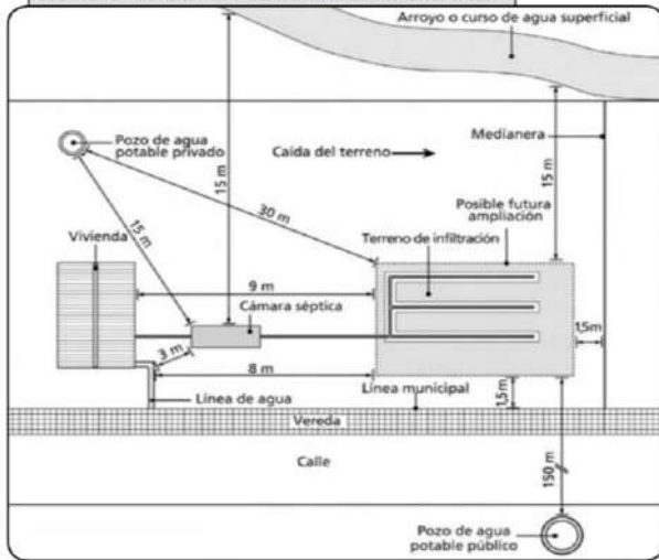
FIGURA 5 - UBICACIÓN Y DISTANCIAS RECOMENDABLES
