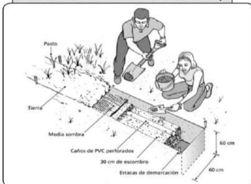
FIGURA 14 - CONSTRUCCIÓN DEL TERRENO DE INFILTRACIÓN - Zanjas
