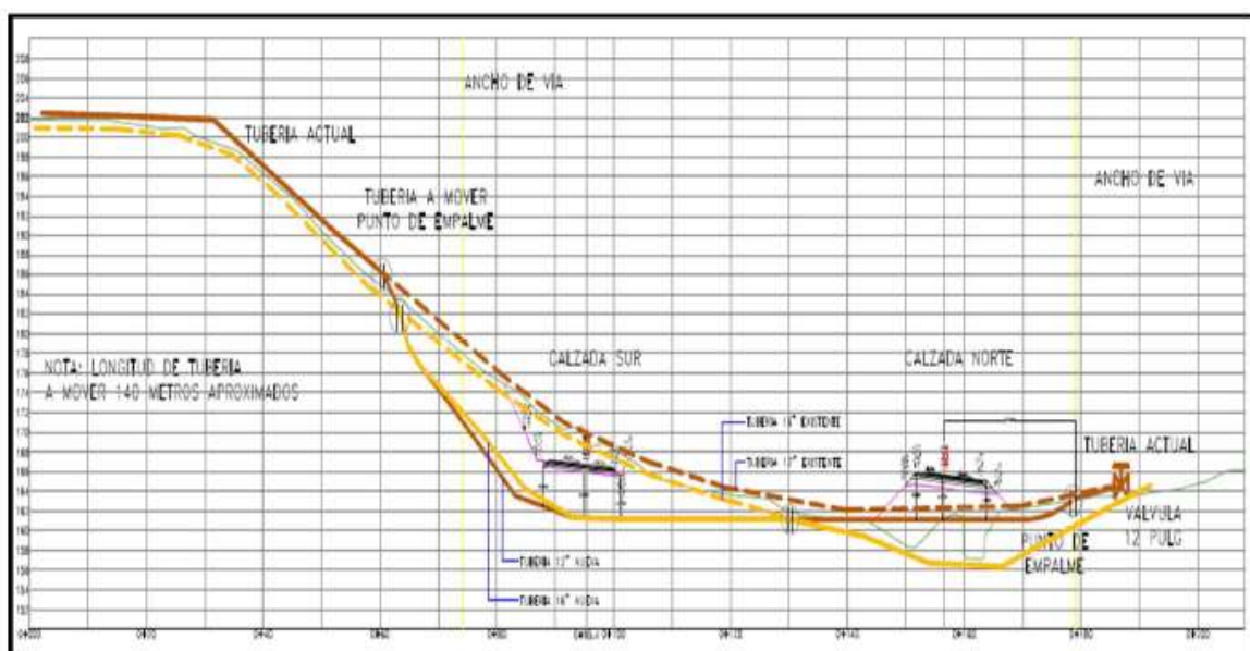
Ilustración 7 Variantes verticales
