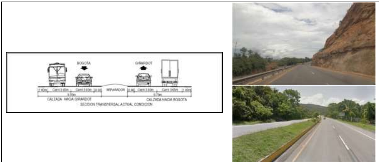
Figura 2 UF 1 Vista General y Sección Transversal Típica, PR25+000 y PR35+000
