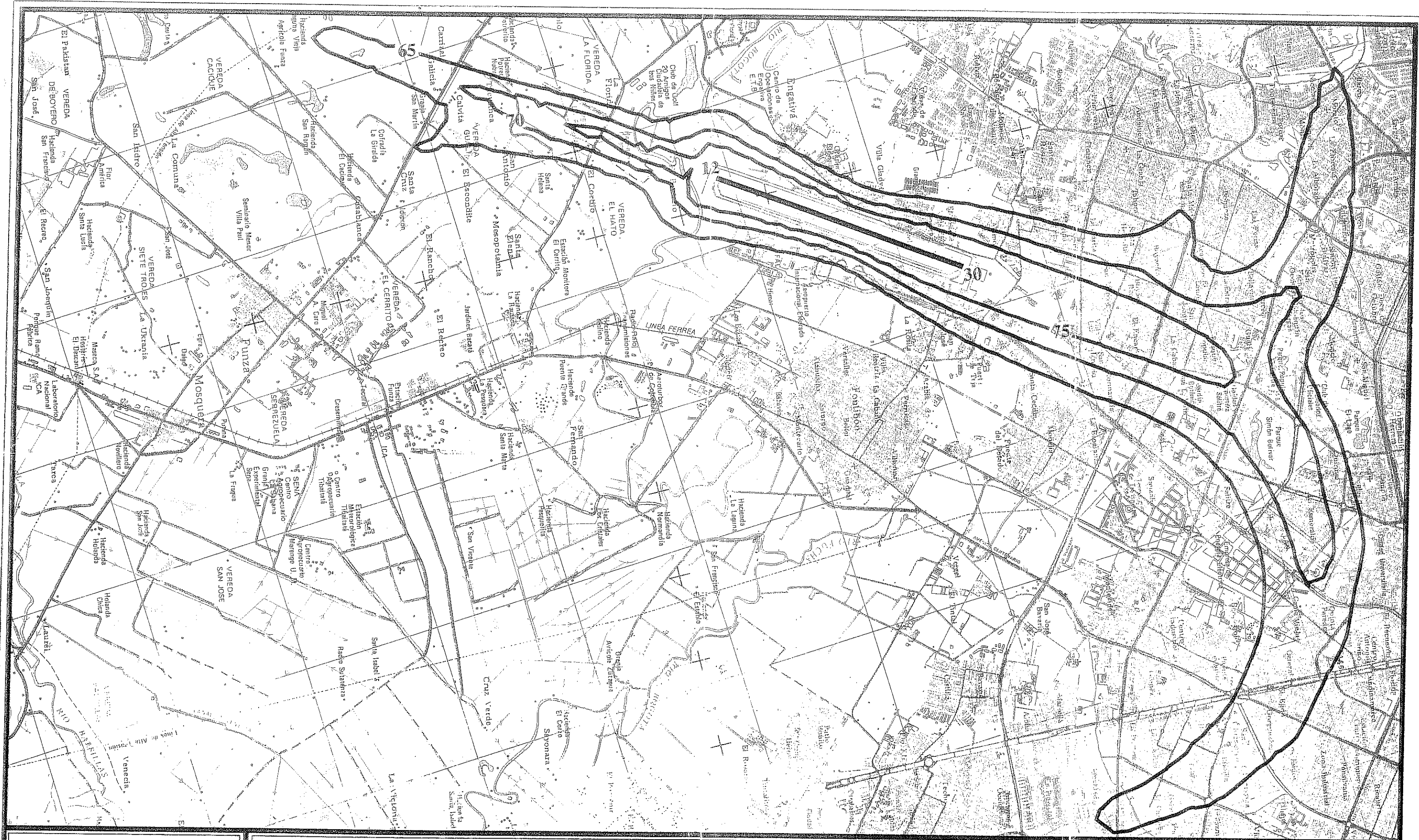
FIGURA 4.32 Modelaje de Niveles de Ruido Efecto de Flota Actual Para Una Sola Pista en 1.993
