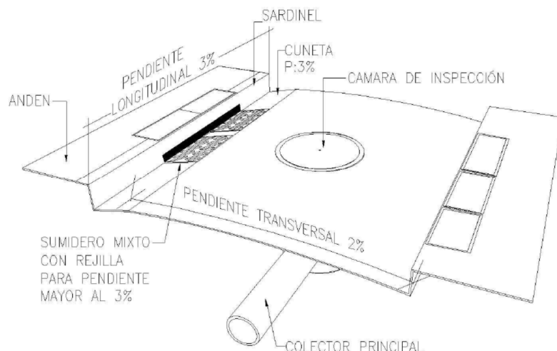
Detalle de drenaje tipo en nuevos viales.
