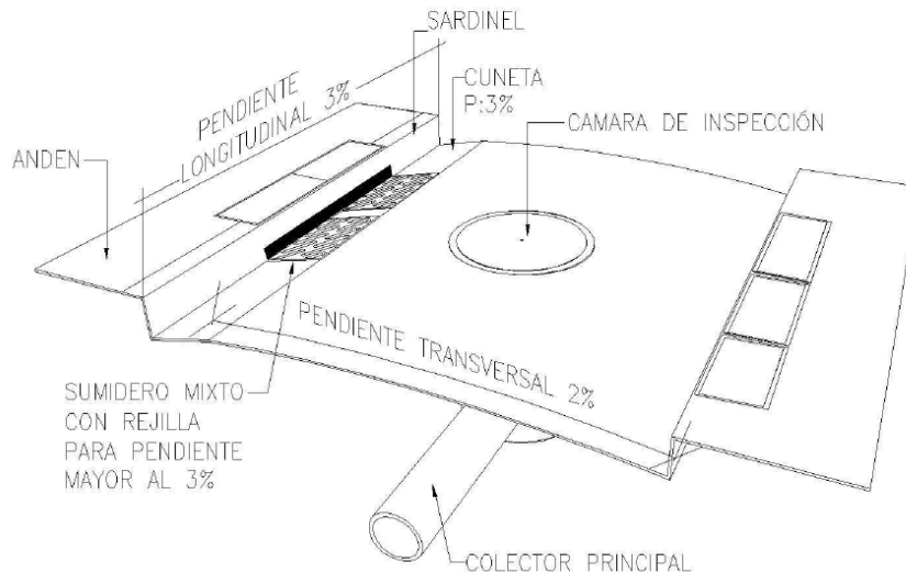
Detalle de drenaje tipo en nuevos viales.
