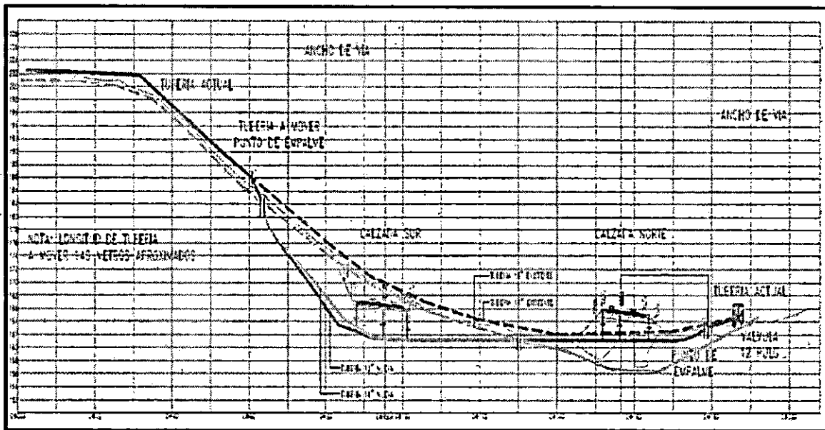
Ilustración 7 Variantes verticales
