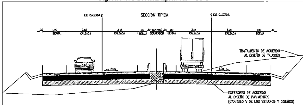
Figura No. 5 Sección típica vía – UF-3
