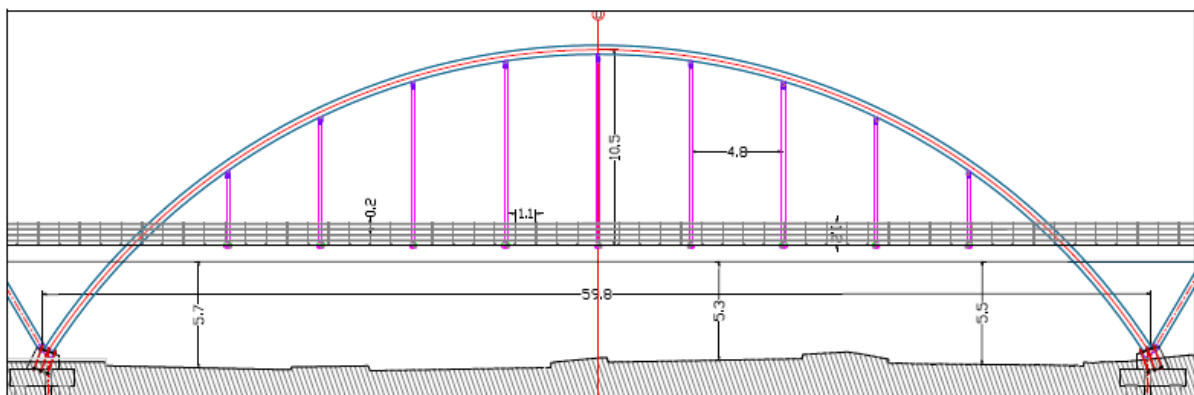
Ilustración 2. Vista Longitudinal Puente Peatonal “Camilo Torres”
