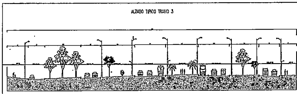
Alzado Típico Tramo 3
