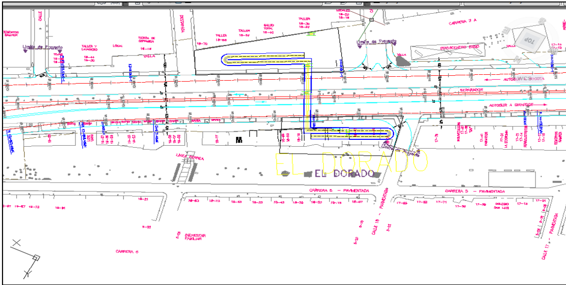
Gráfico de Implantación Puente Peatonal El Dorado – Abscisa K3+995
