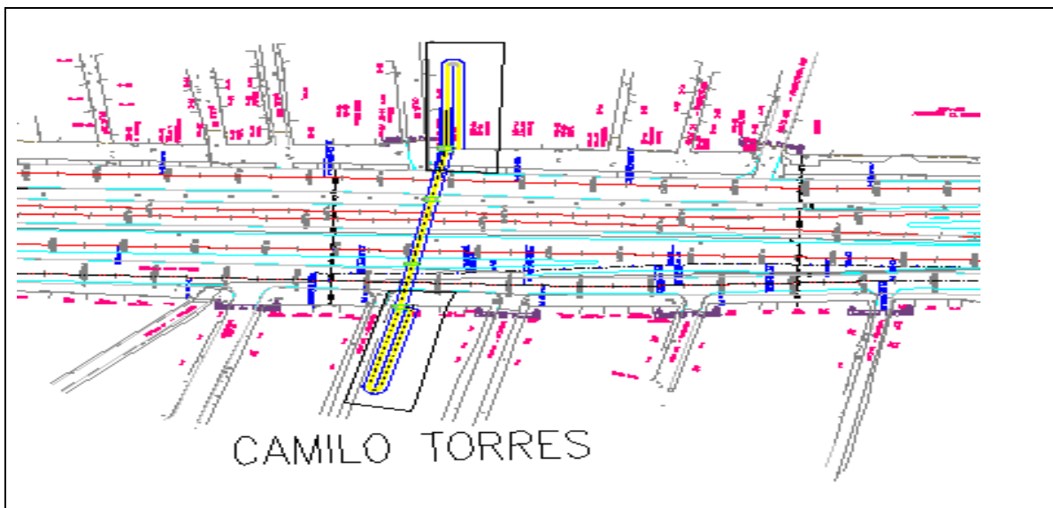
Gráfico De Implantación Puente Peatonal Camilo Torres - Abscisa K3+385
