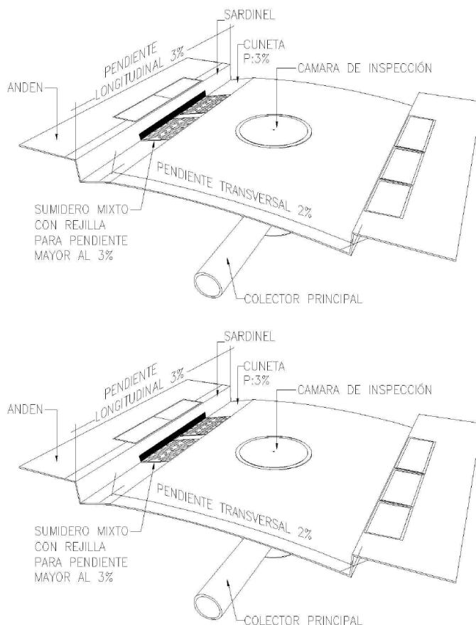
Detalle de drenaje tipo en nuevos viales.
